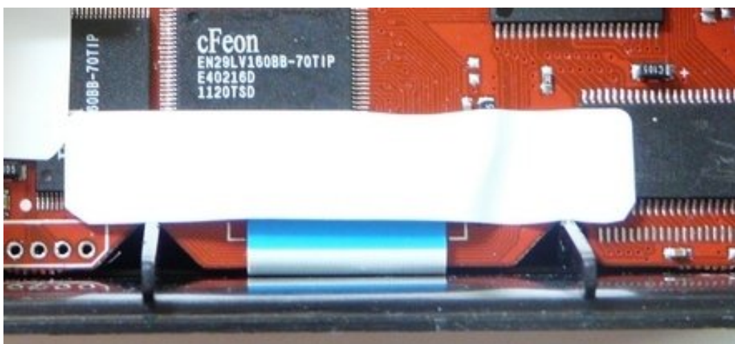
Slika 3. – izgled postavljene plombe, plomba se postavlja preko konektora na način koji onemogućava zamenu fiskalne memorije bez skidanja fiskalne plombe
