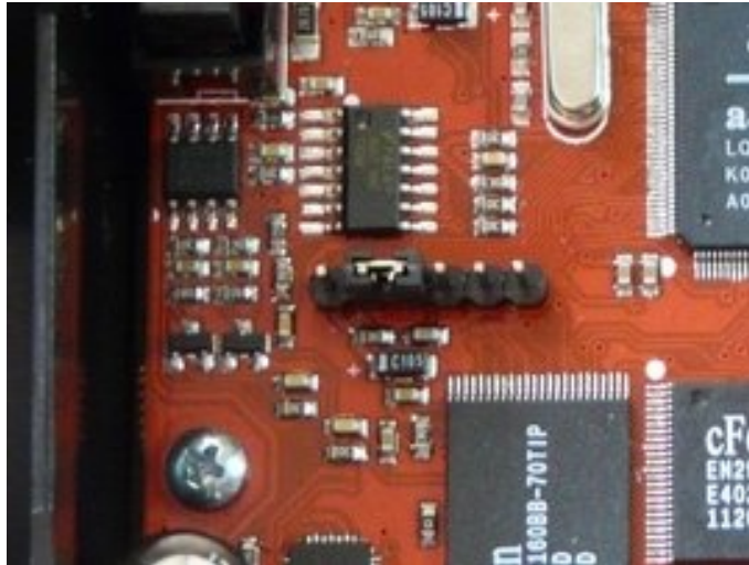
Slika 4. – konektor za programiranje sa zaštitnim kratkospojnikom
