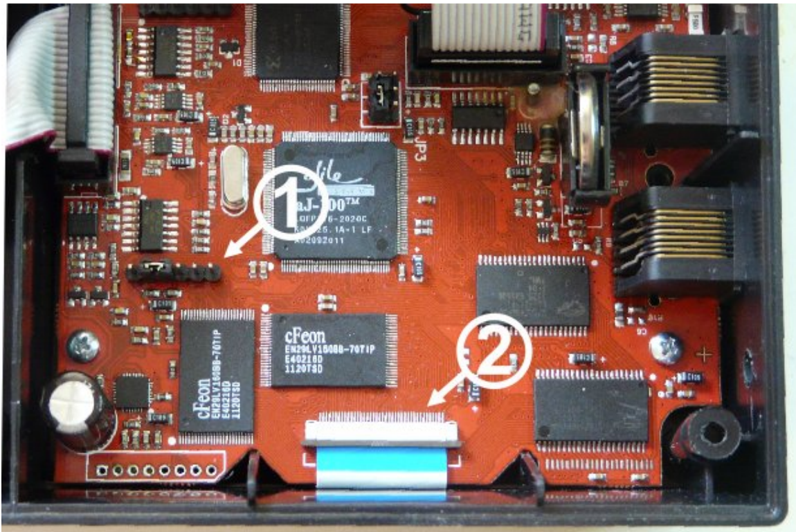
Slika 1. – Izgled ploče i mesto postavljanja plombi
